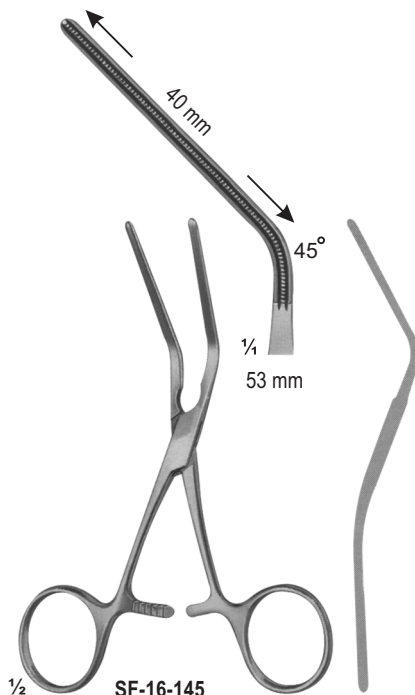
SF-16-145 DE-BAKEY 45° winklig gebogen angled 45° 125 mm
