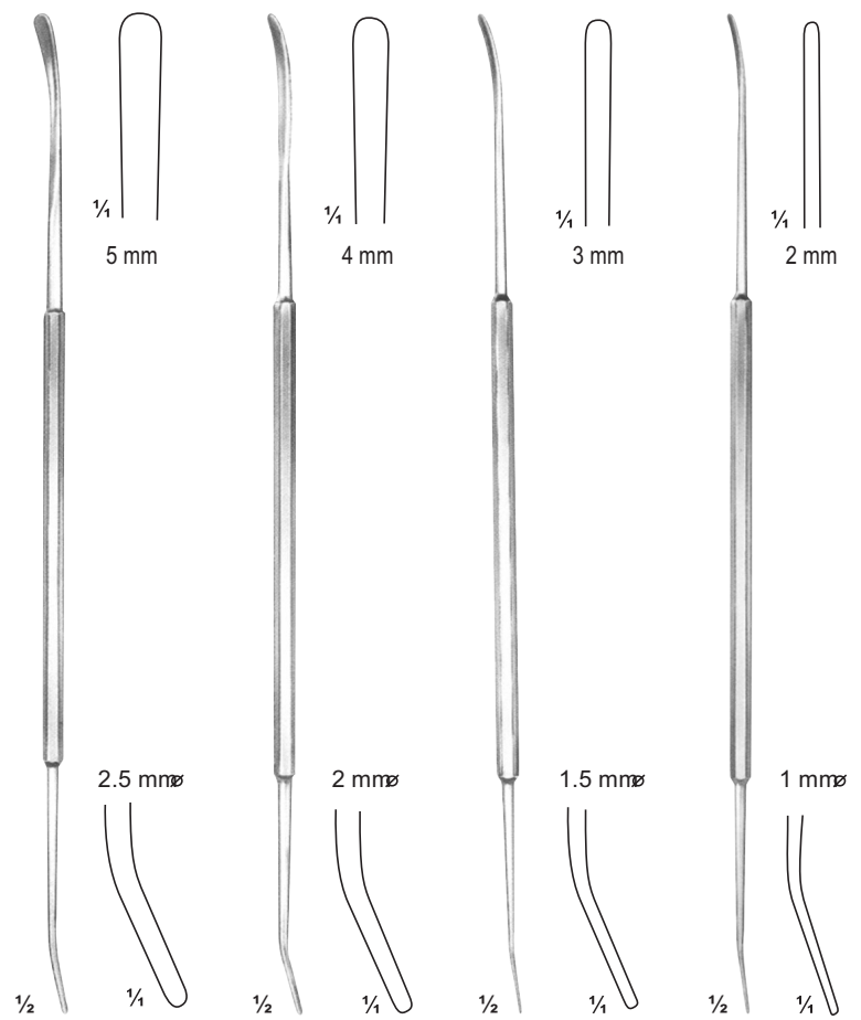
Fig. 1 ROBB SF-16-457 24 cm
